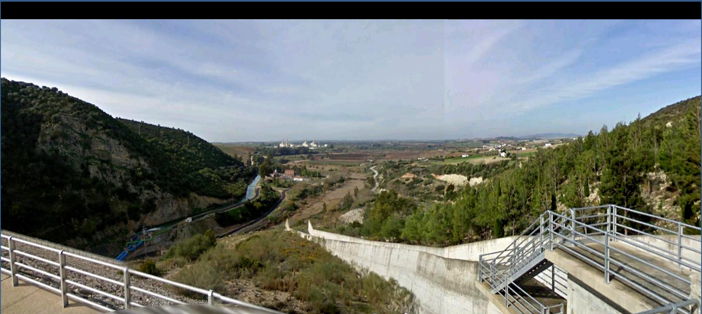
Relieves Jurásicos desde coronación del Embalse del Guadalcacín, SW Hoja de Arcos de La Frontera
