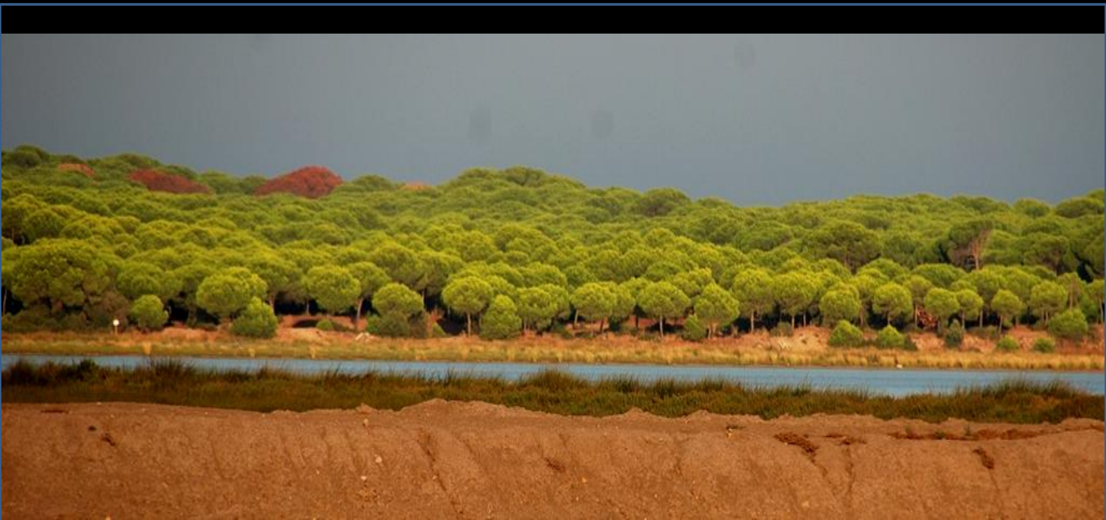
En el Holoceno al N de Bonanza. N Hoja de Sanlúcar de Barrameda. (por chaolopez-google)
